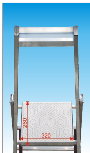
Piattaforma EXTRALARGE in alluminio per la massima stabilità e sicurezza
