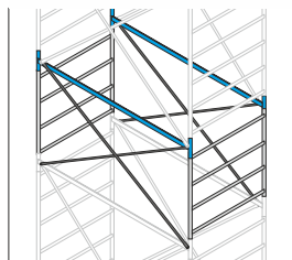
Campata a n°4 gradini EXP-HD CAMP
