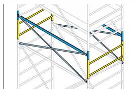
Mezza Campata a n°2 gradini EXP-HD1/2CA
