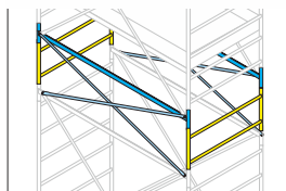
Mezza Campata a n°2 gradini PSP 1/2 CAM
