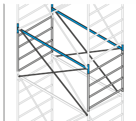
Campata a n°4 gradini PSP CAMPATA
