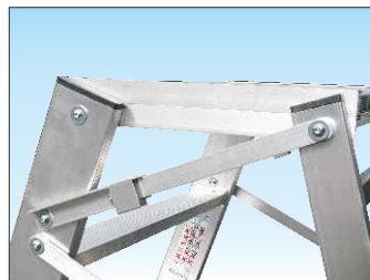
Dispositivo di bloccaggio automatico di sicurezza anti-apertura e anti-chiusura
