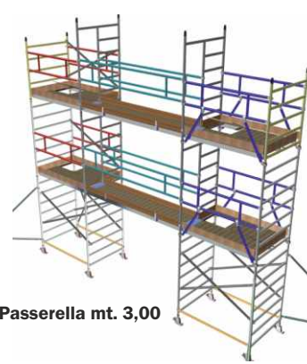
Passerella con superficie in lamiera mandrolata di alluminio
