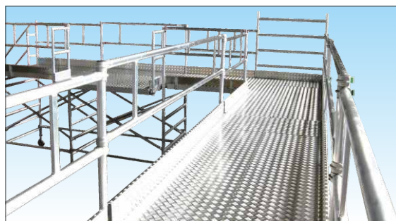
Passerella con superficie in lamiera mandrolata di alluminio
