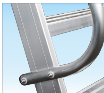
Corrimano realizzato in tubo tondo Ø 32 mm. con fissaggio regolabile
