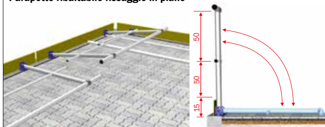
Parapetto ribaltabile fissaggio in piano
