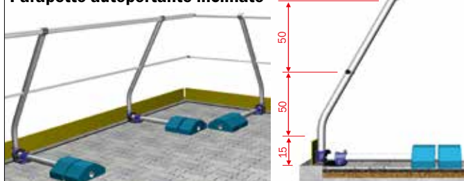
Parapetto autoportante inclinato
