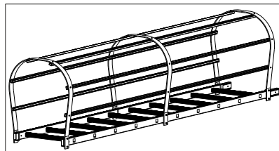
[Fig. 5] - APPLICAZIONE DEI CORRIMANI D'USCITA e DEGLI ANELLI SU MODULO TERMINALE
